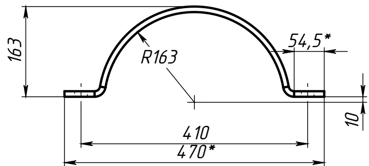
Поз.4 (Полухомут)
